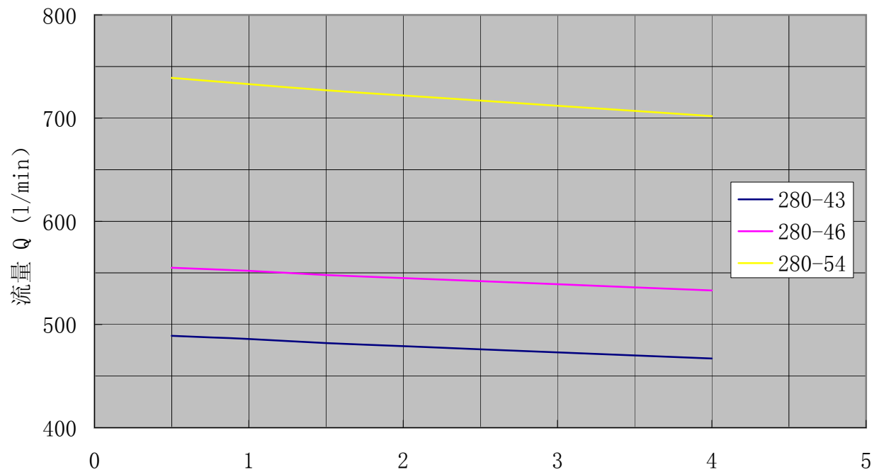
SN280性能曲线 转速:2900r/min 粘度:75mm 2 /s
