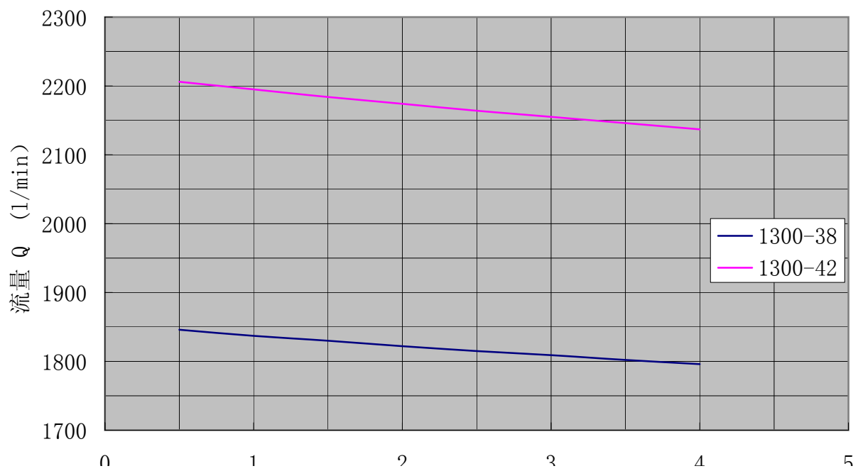
SN1300性能曲线 转速:2900r/min 粘度:75mm 2 /s
