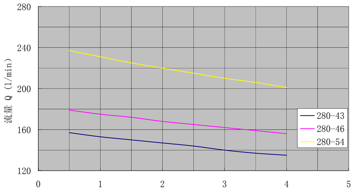
SN280性能曲线 转速:950r/min 粘度:75mm 2 /s
