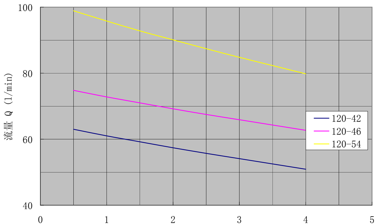
SN120 性能曲线 转速:950r/min 粘度:75mm 2 /s
