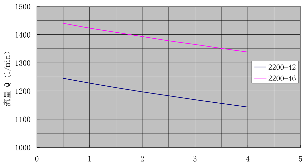
SN2200 性能曲线 转速:950r/min 粘度:75mm 2 /s
