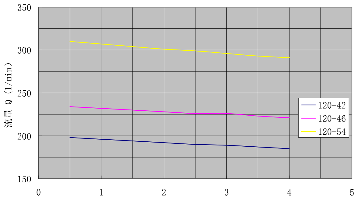
SN120性能曲线 转速:2900r/min 粘度:75mm 2 /s
