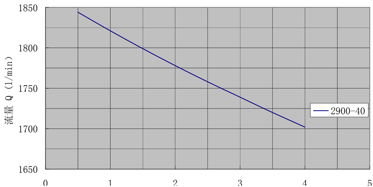
SN 2900性能曲线 转速:950r/min 粘度:75mm 2 /s
