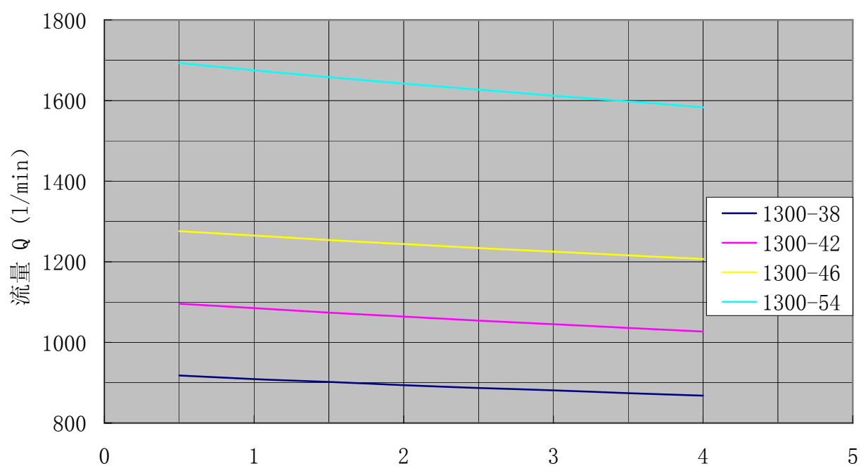
SN1300性能曲线 转速:1450r/min 粘度:75mm 2 /s
