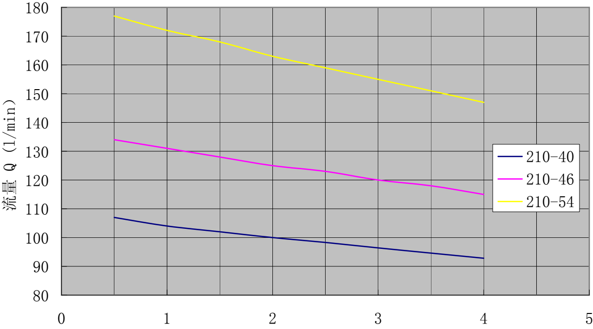
SN210性能曲线 转速:950r/min 粘度:75mm 2 /s
