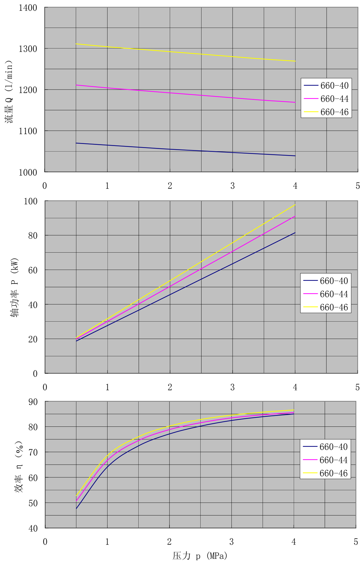
SN660 性能曲线 转速:2900r/min 粘度:75mm 2 /s
