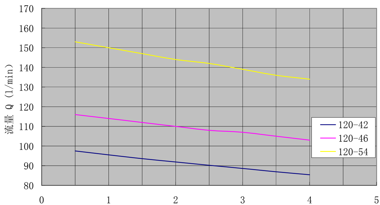
SN120性能曲线 转速:1450r/min 粘度:75mm 2 /s
