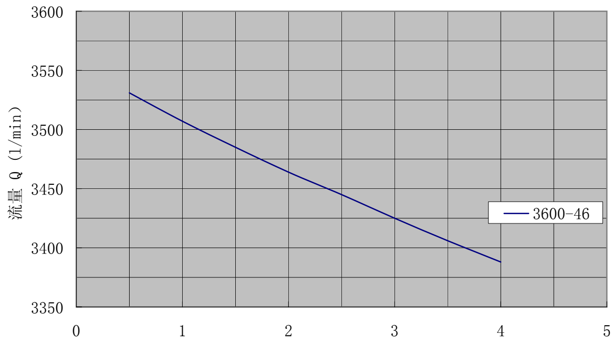
SN3600性能曲线
