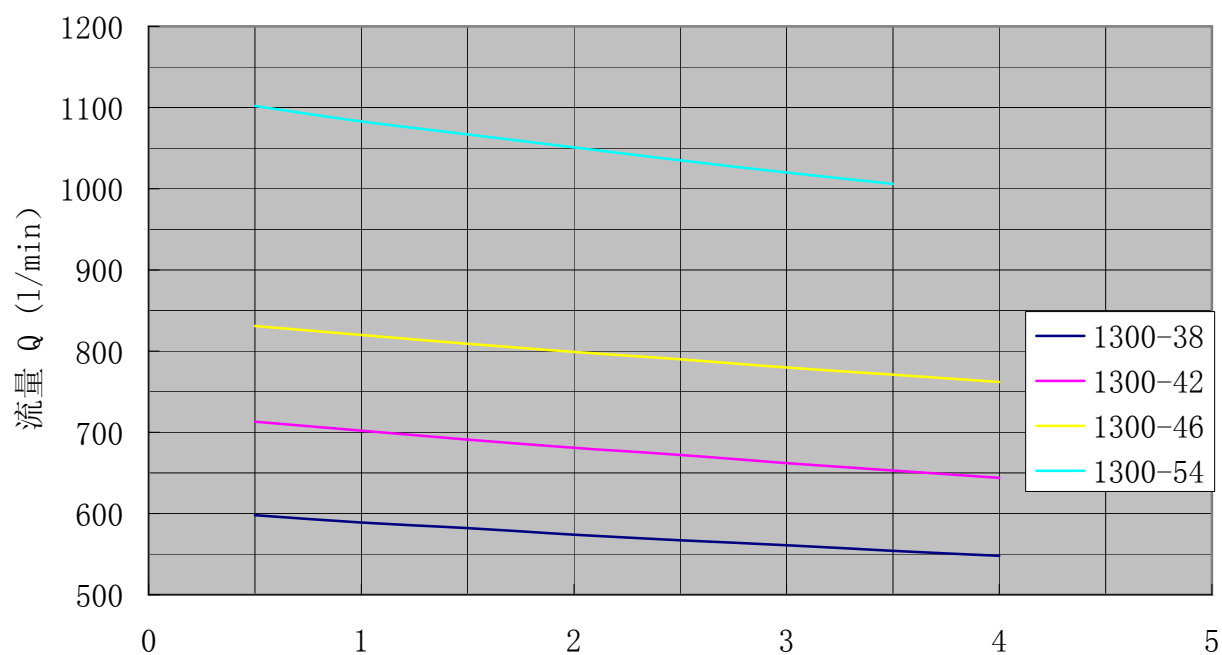
SN1300性能曲线 转速:950r/min 粘度:75mm 2 /s
