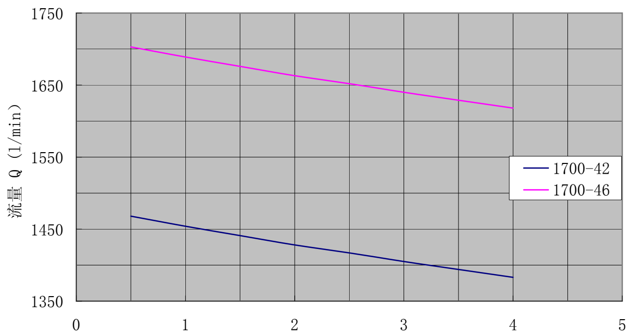
SN1700性能曲线 转速:1450r/min 粘度:75mm 2 /s
