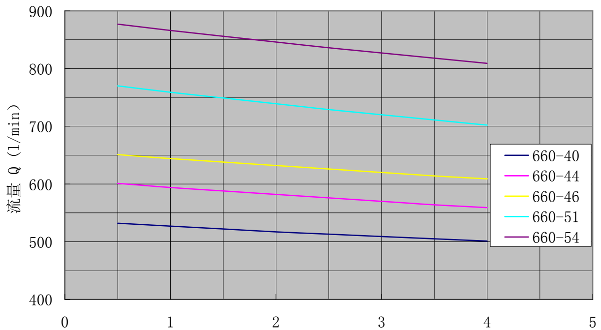
SN660性能曲线 转速:1450r/min 粘度:75mm 2 /s
