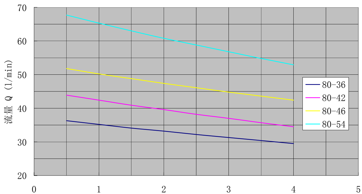
SN80 性能曲线 转速:950r/min 粘度:75mm 2 /s
