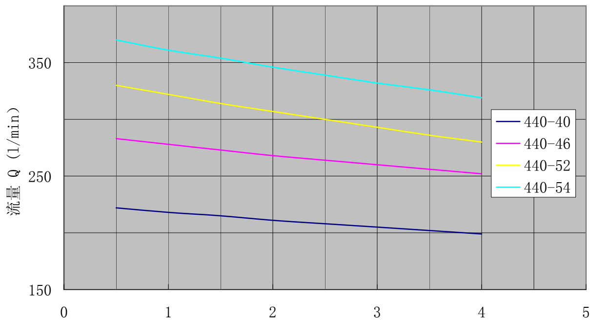
SN440性能曲线 转速:950r/min 粘度:75mm 2 /s
