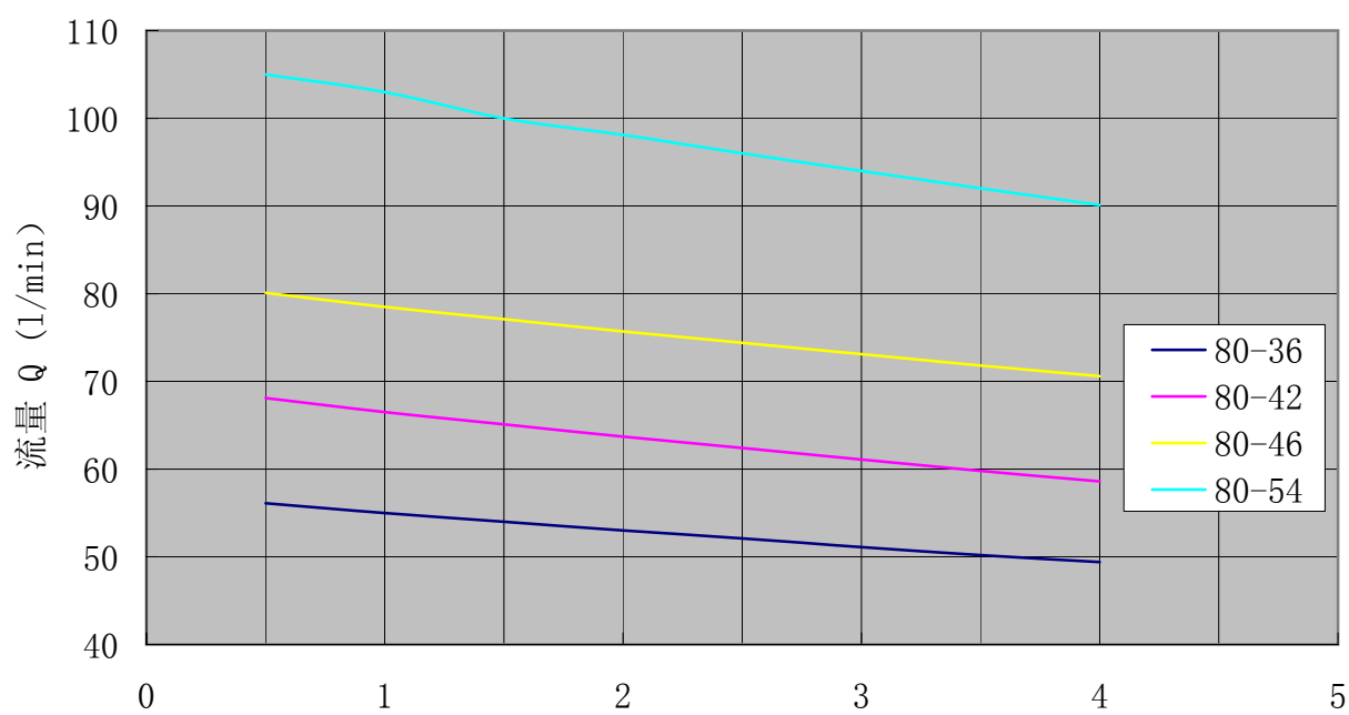
SN80性能曲线 转速:1450r/min 粘度:75mm 2 /s
