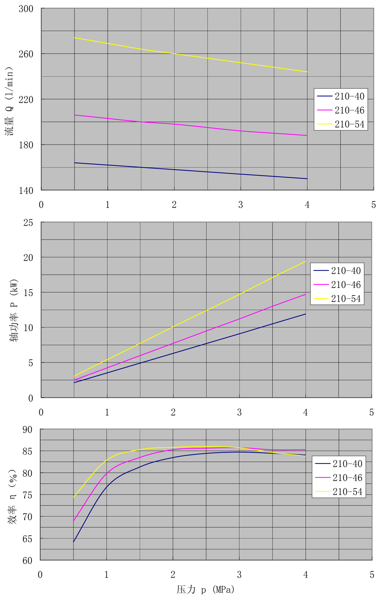
SN210性能曲线 转速:1450r/min 粘度:75mm 2 /s
