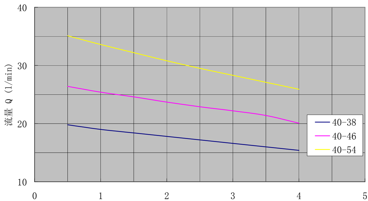
SN40性能曲线 转速:950r/min 粘度:75mm 2 /s
