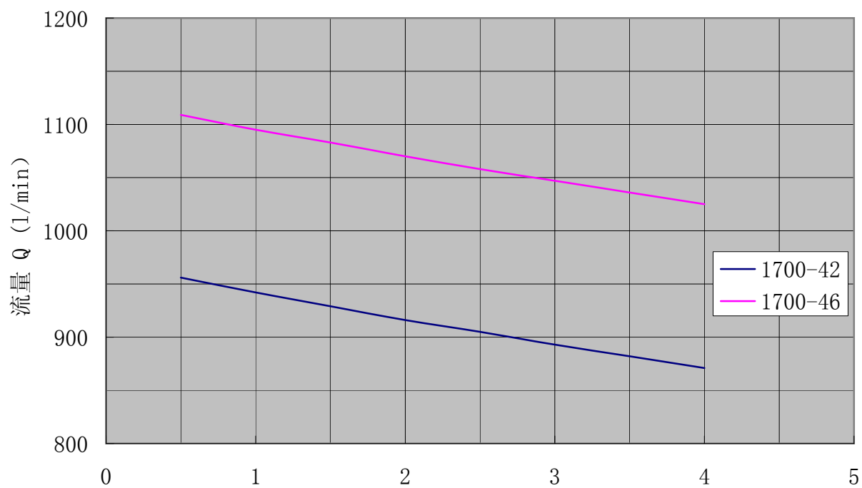
SN1700性能曲线
