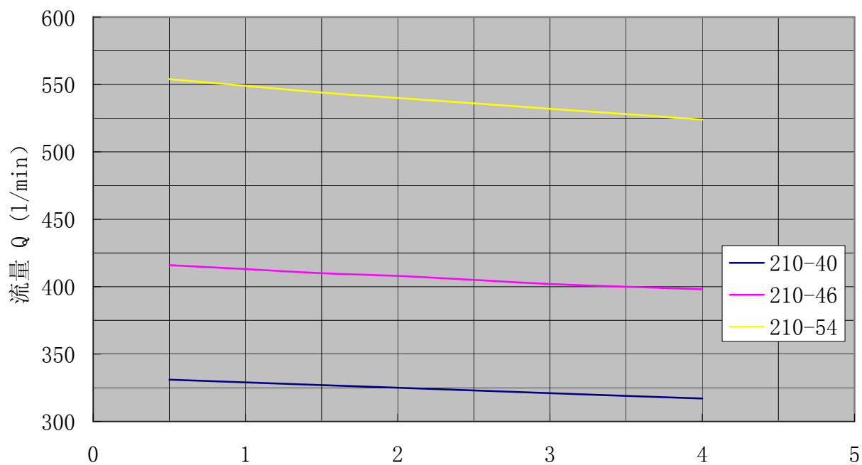
SN210性能曲线 转速:2900r/min 粘度:75mm 2 /s
