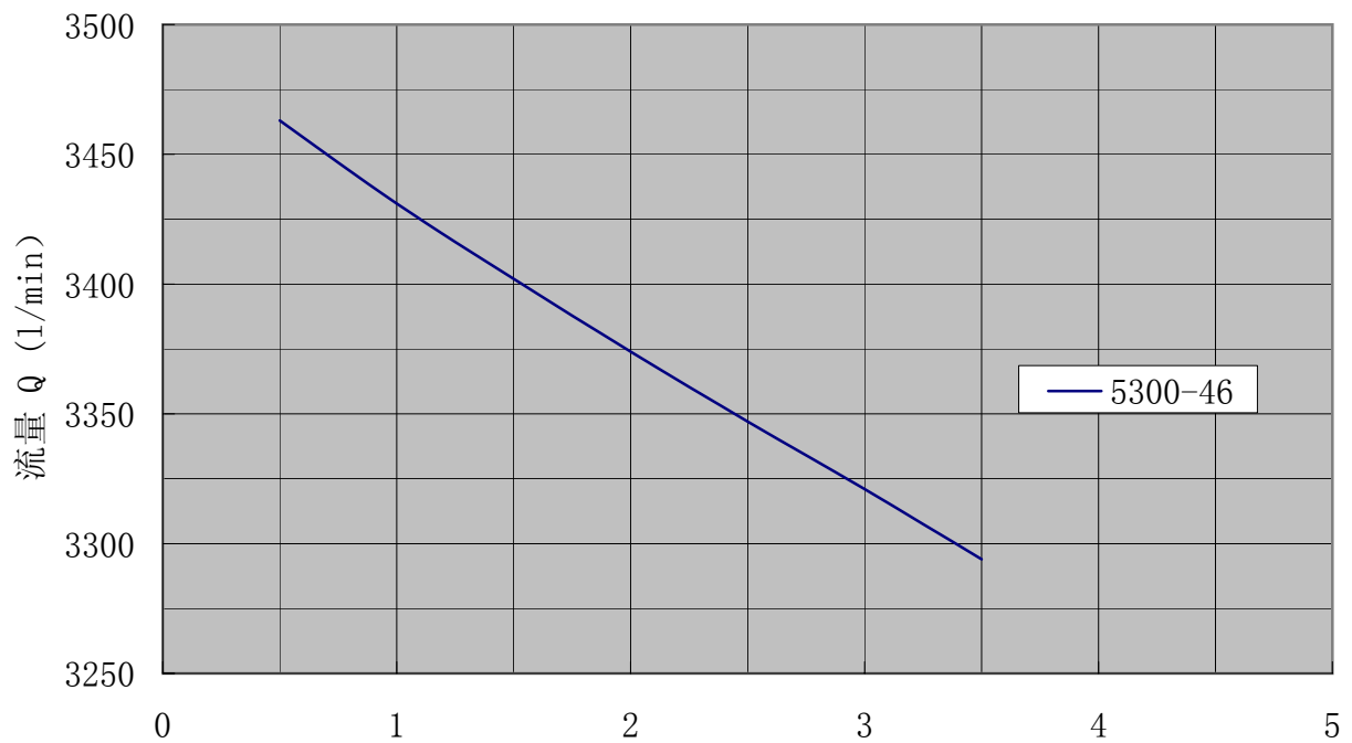
SN5300性能曲线 转速:950r/min 粘度:75mm 2 /s
