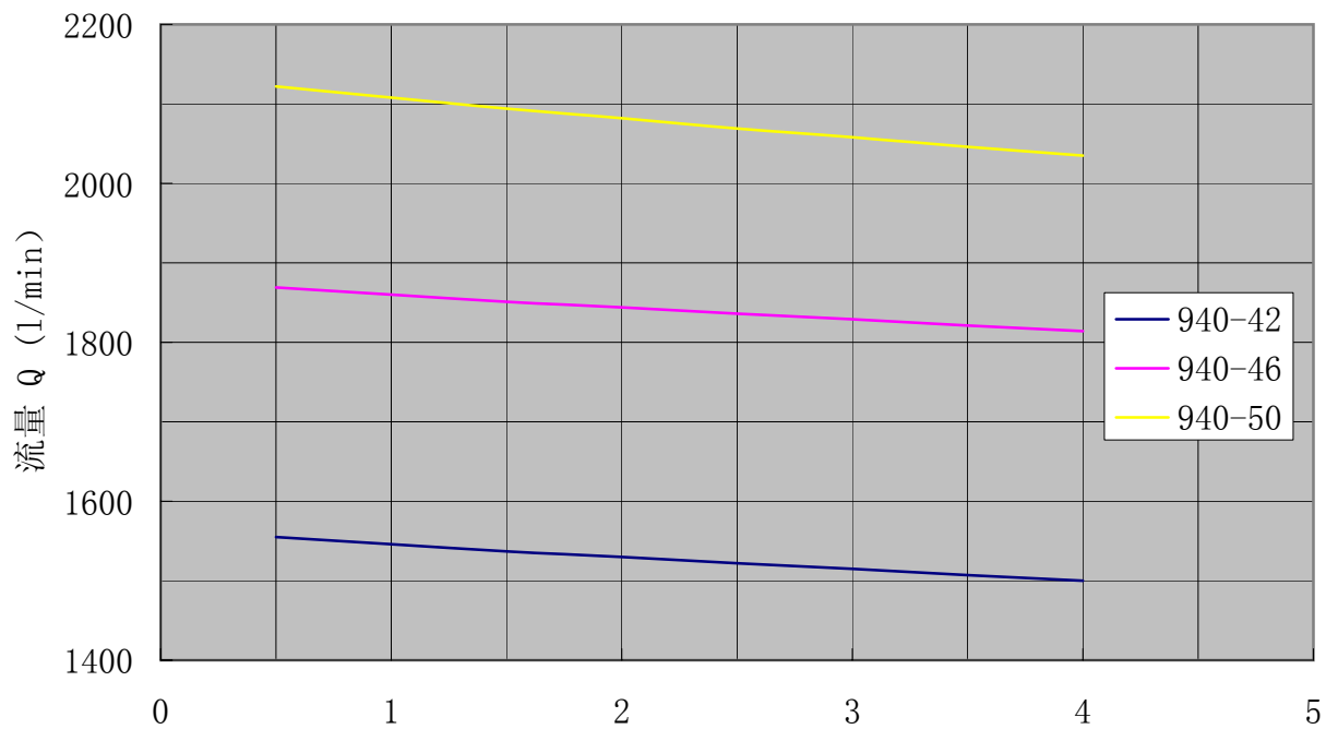
SN940性能曲线 转速:2900r/min 粘度:75mm 2 /s
