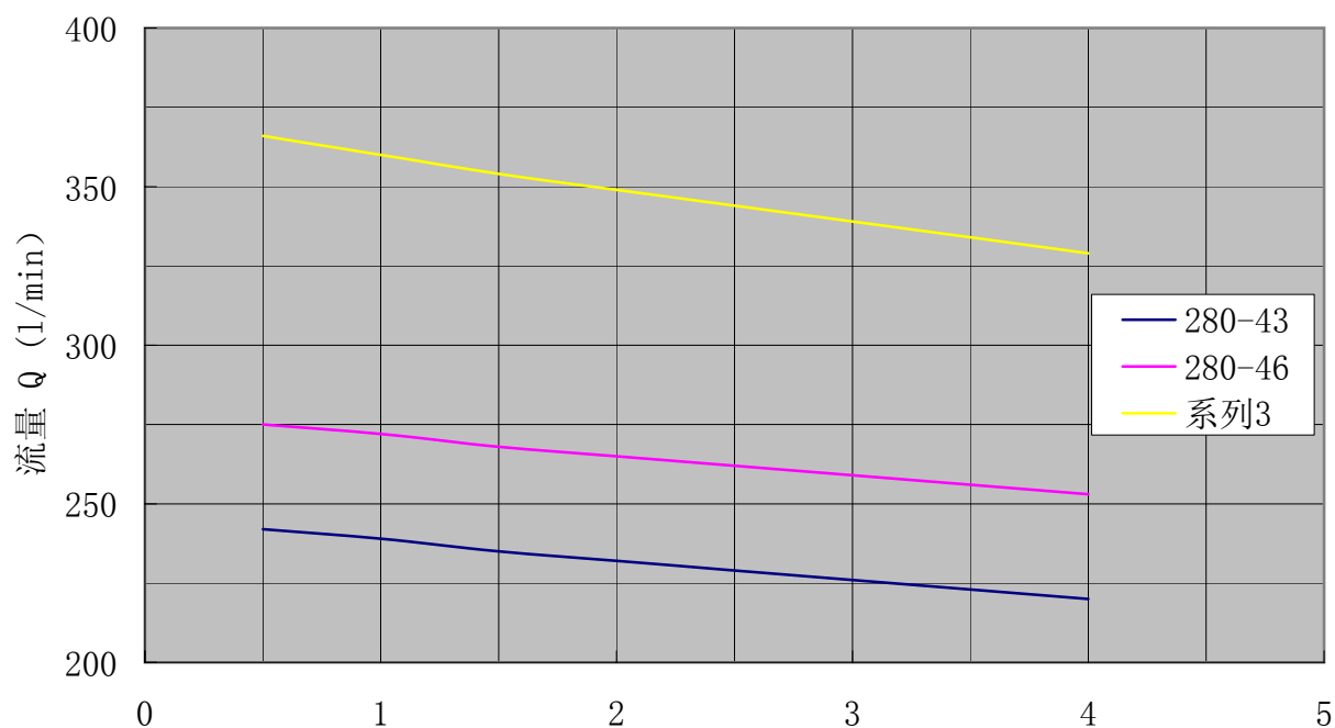
SN280性能曲线 转速:1450r/min 粘度:75mm 2 /s
