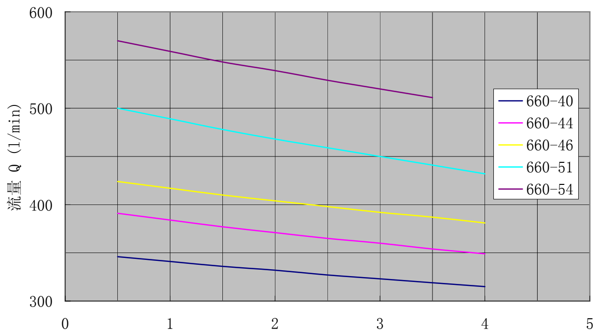
SN660性能曲线 转速:950r/min 粘度:75mm 2 /s
