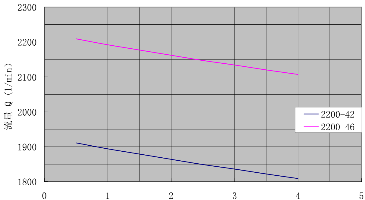
SN2200性能曲线
