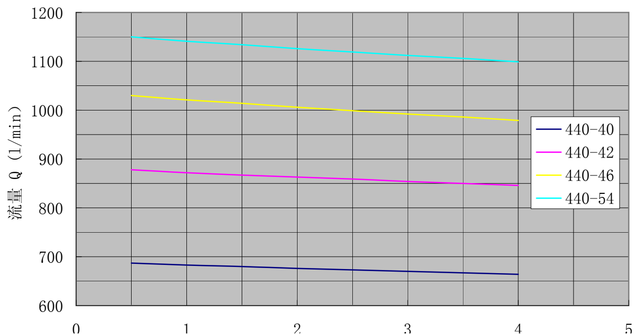
SN440性能曲线 转速:2900r/min 粘度:75mm 2 /s
