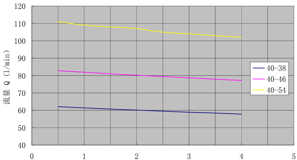
SN40性能曲线 转速:2900r/min 粘度:75mm 2 /s
