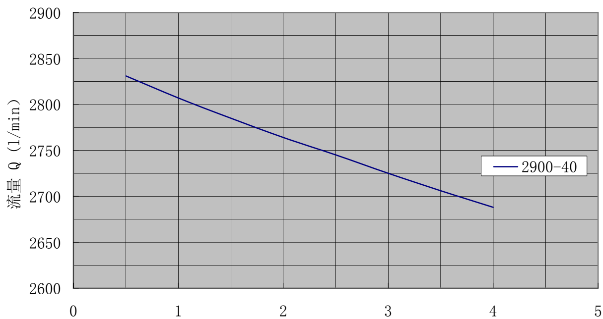
SN2900性能曲线
