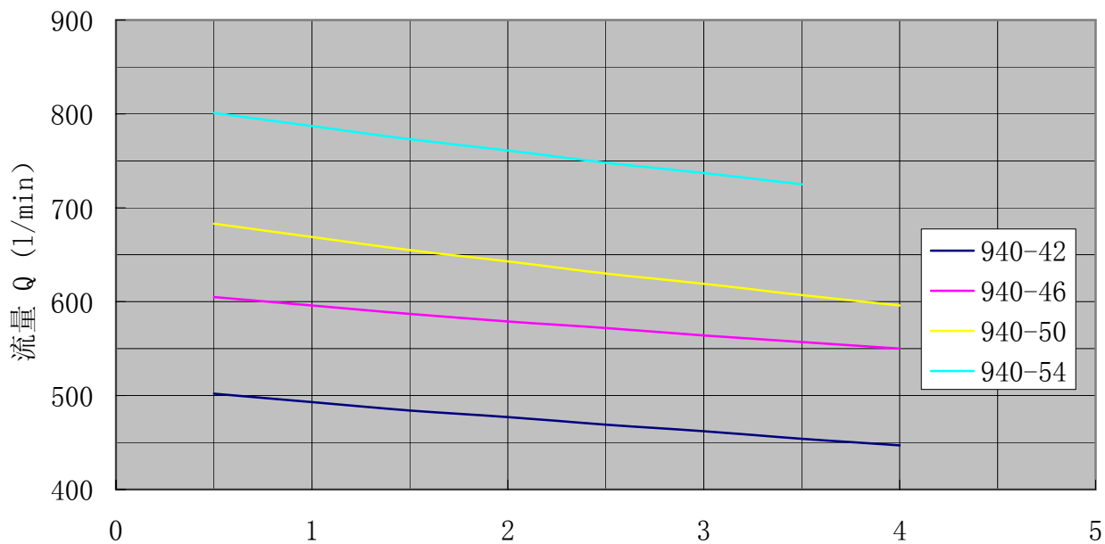
SN940性能曲线 转速:950r/min 粘度:75mm 2 /s
